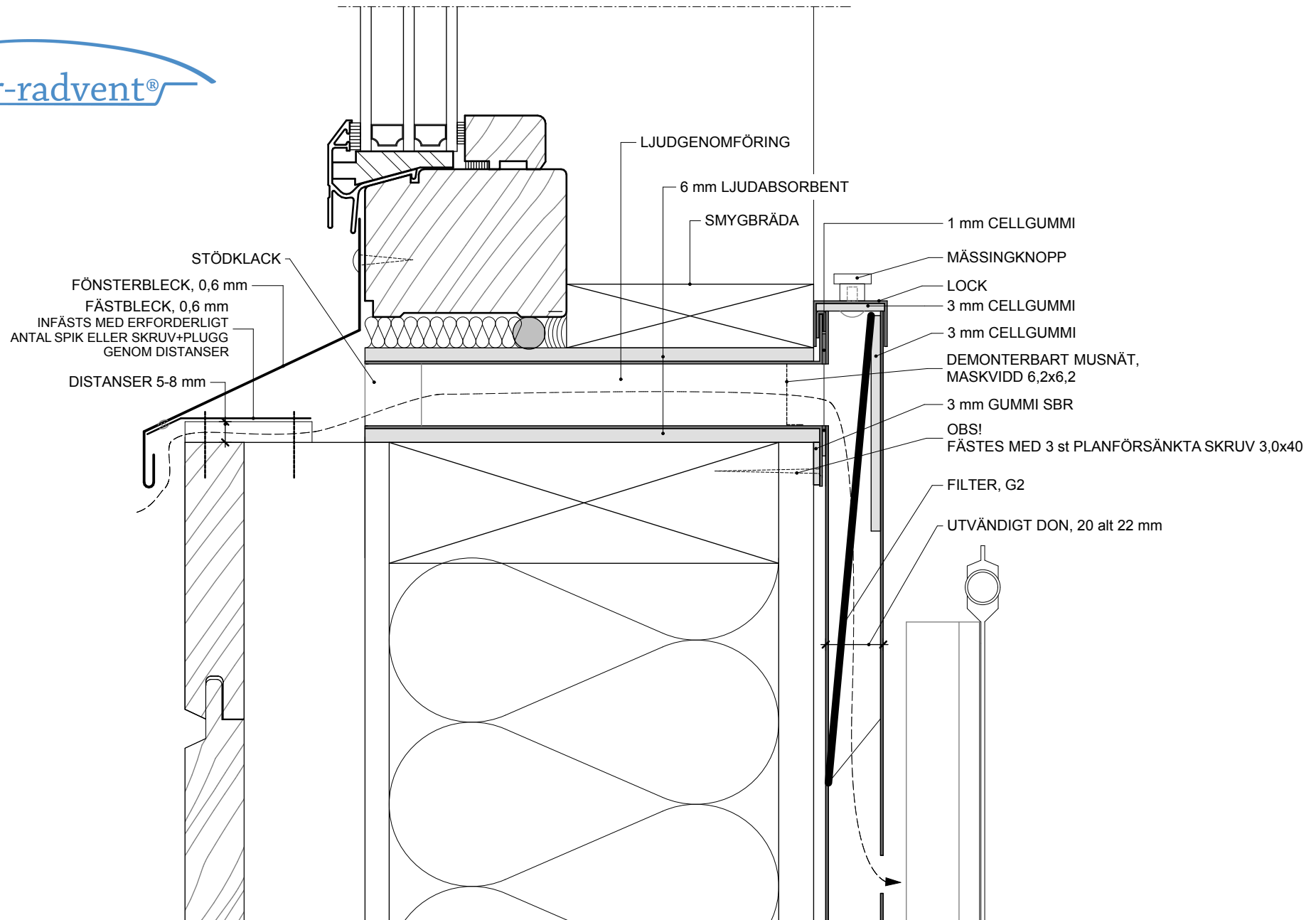
SEKTION GENOM TRÄFASAD - LJUDKLASSAT UTFÖRANDE
