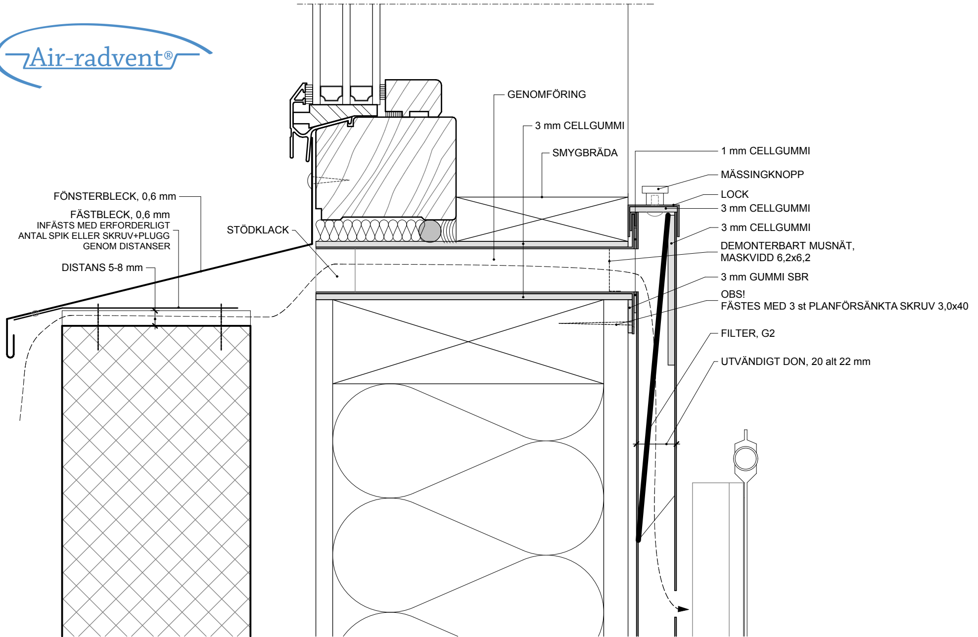
SEKTION GENOM PREFAB-FASAD
